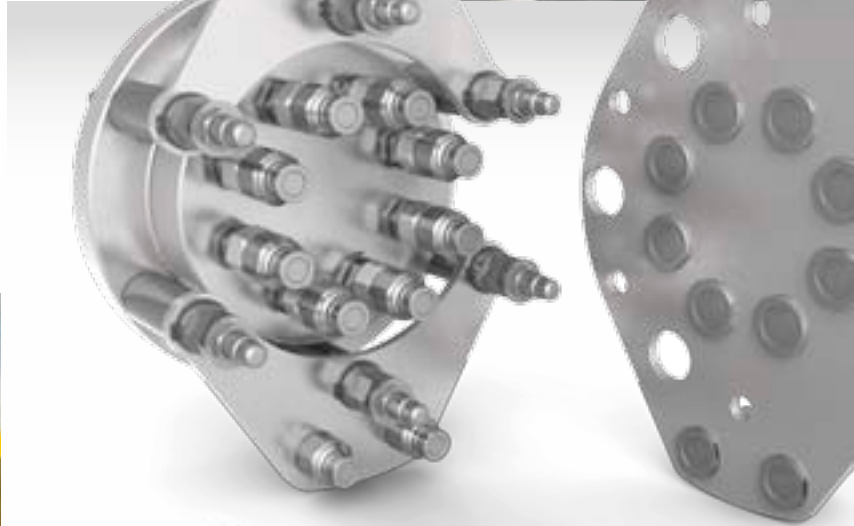
YouTube 应用于造纸机械的多路连接接头 手动连接板上装有8套665系列接头和4套565系列接头。连接板采用不锈钢制造
